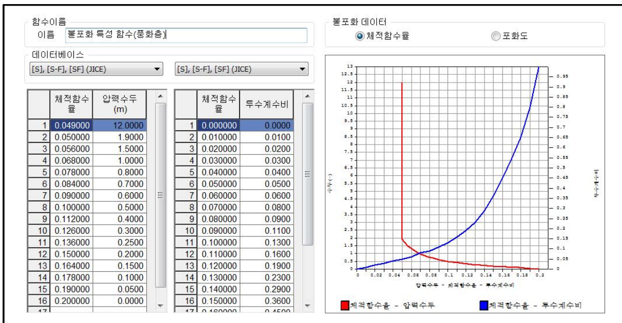
【그림 20.15】 압력수두-체적함수(포화도)-투수계수비 함수
