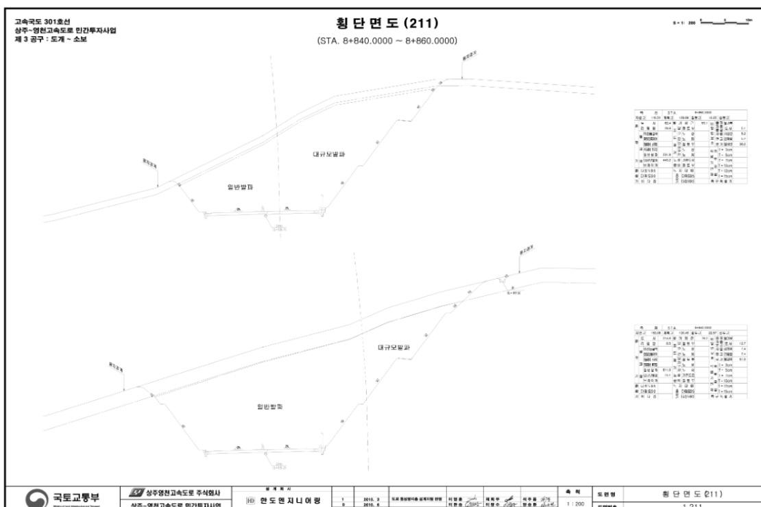
【그림 20.4】 표준횡단면도
